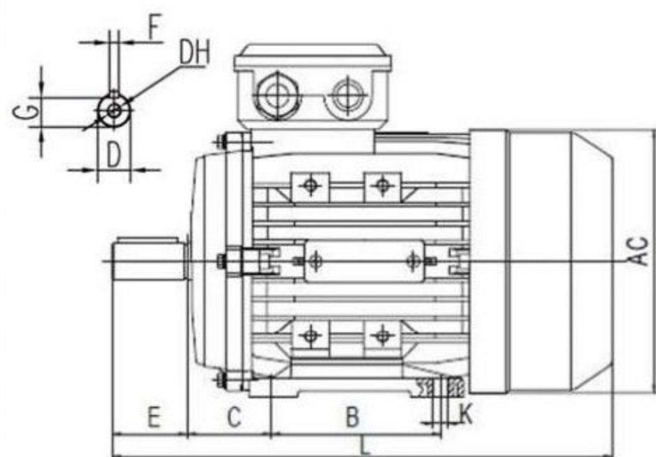
B3 IM 1001
