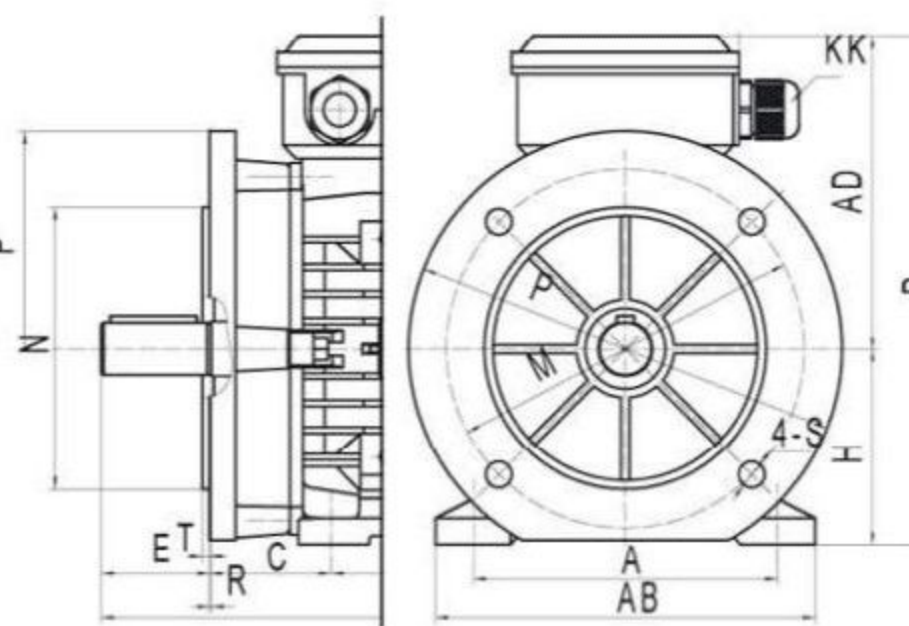
B35 IM 2001
