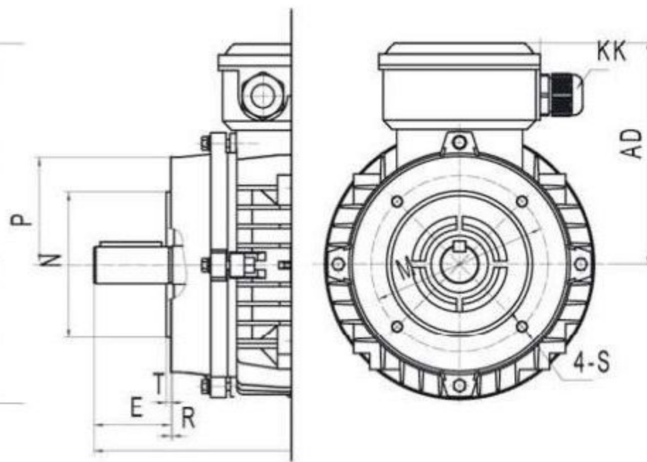
B14 IM 3601
